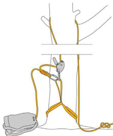
Fig. 5 - Ancoraggio della fune con dispositivo passante
